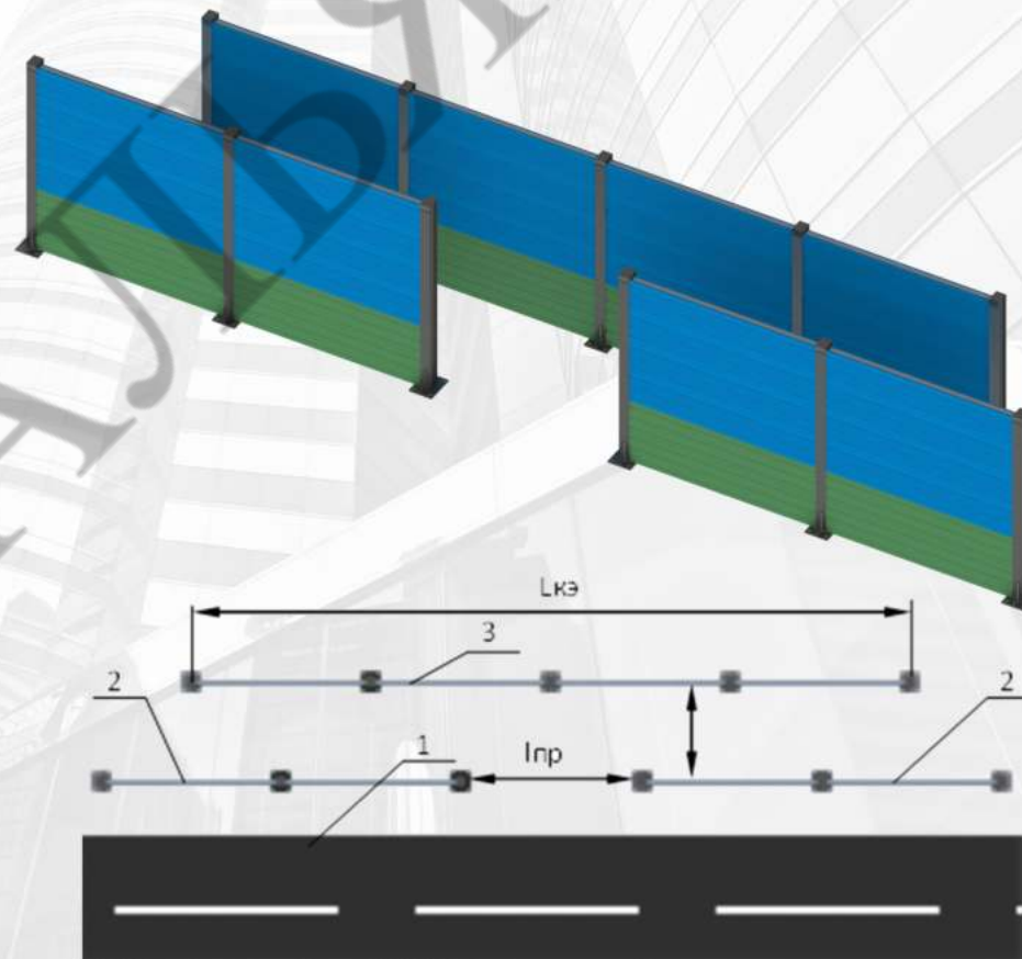
1 – дорога; 2 – экран; 3 – контр-экран. Длина контр-экрана ( L_{кэ} ) должна составлять не менее l_{пр}+4d
